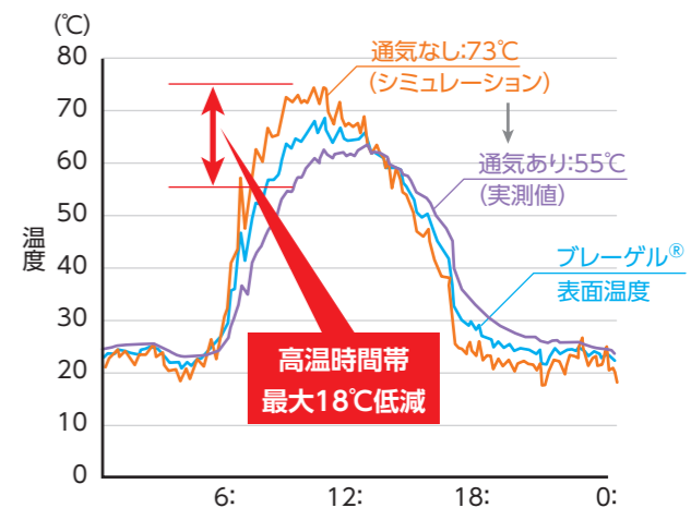
通気なし・ありの温度比較
