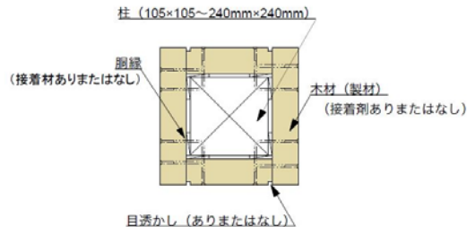
[胴縁ありの場合]
