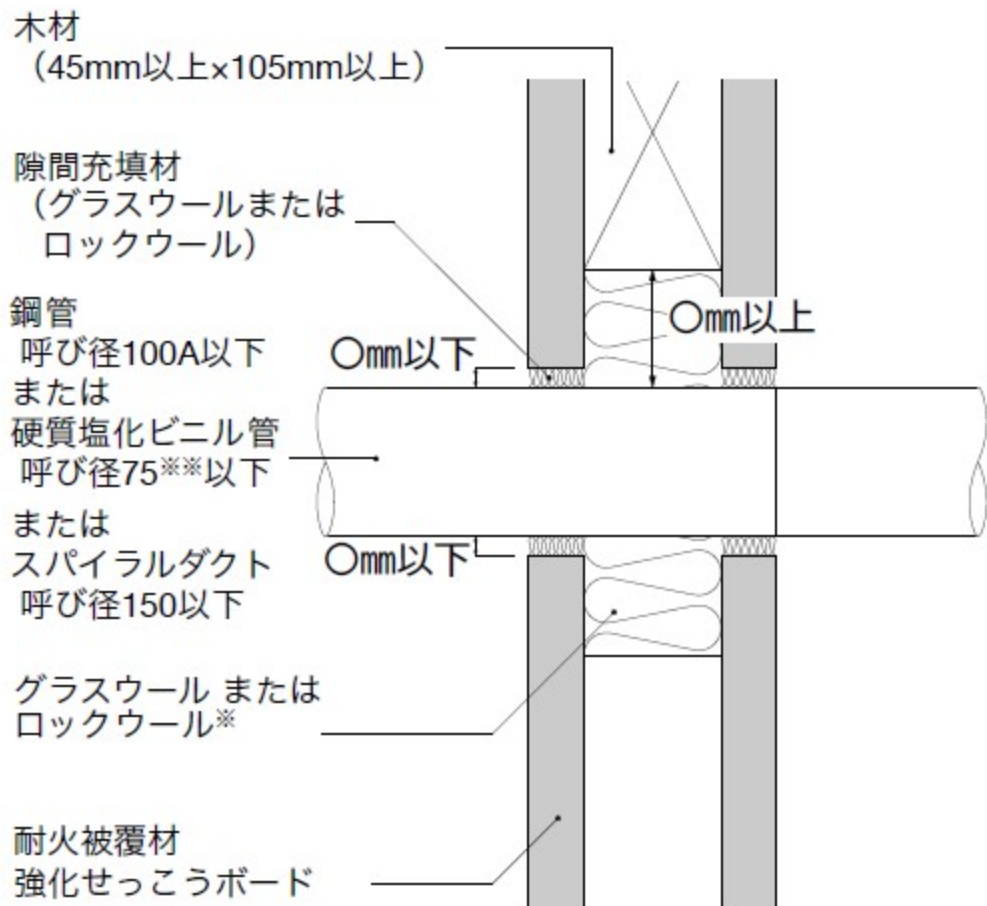
鉛直断面
